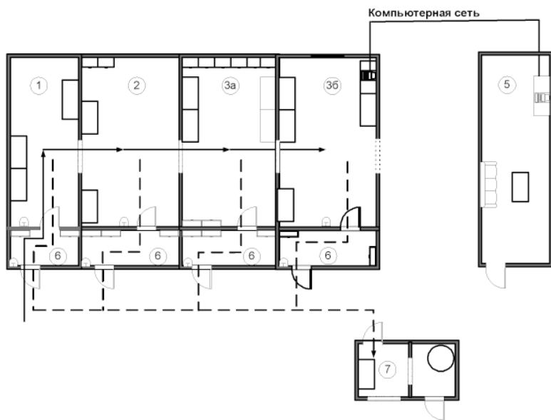
Рис.2. Рекомендуемые схемы размещения помещений (рабочих зон) лаборатории, использующей МАНК с гибридно-флуоресцентным методом детекции продуктов амплификации (А и Б).
